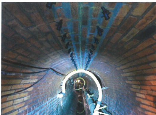
Kanalsanierungen sind eine Spezialität von I+D. Hier: ein alter Hauptsammler in Bocholt
